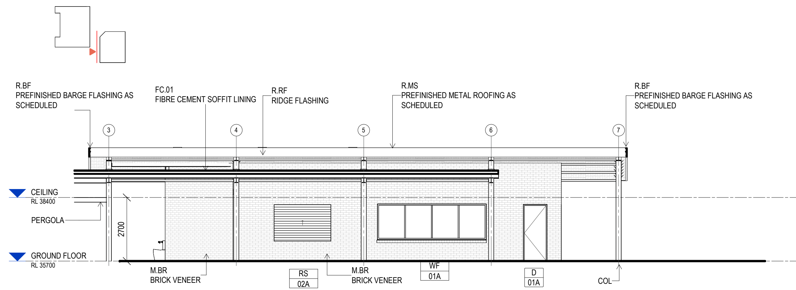
1 ELEVATION WEST Scale: 1 : 100
